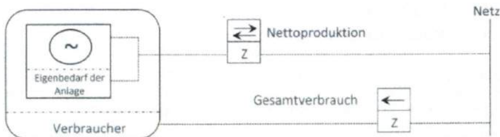
Abbildung 1 : Anordnung der Zähler ohne Eigenverbrauch
