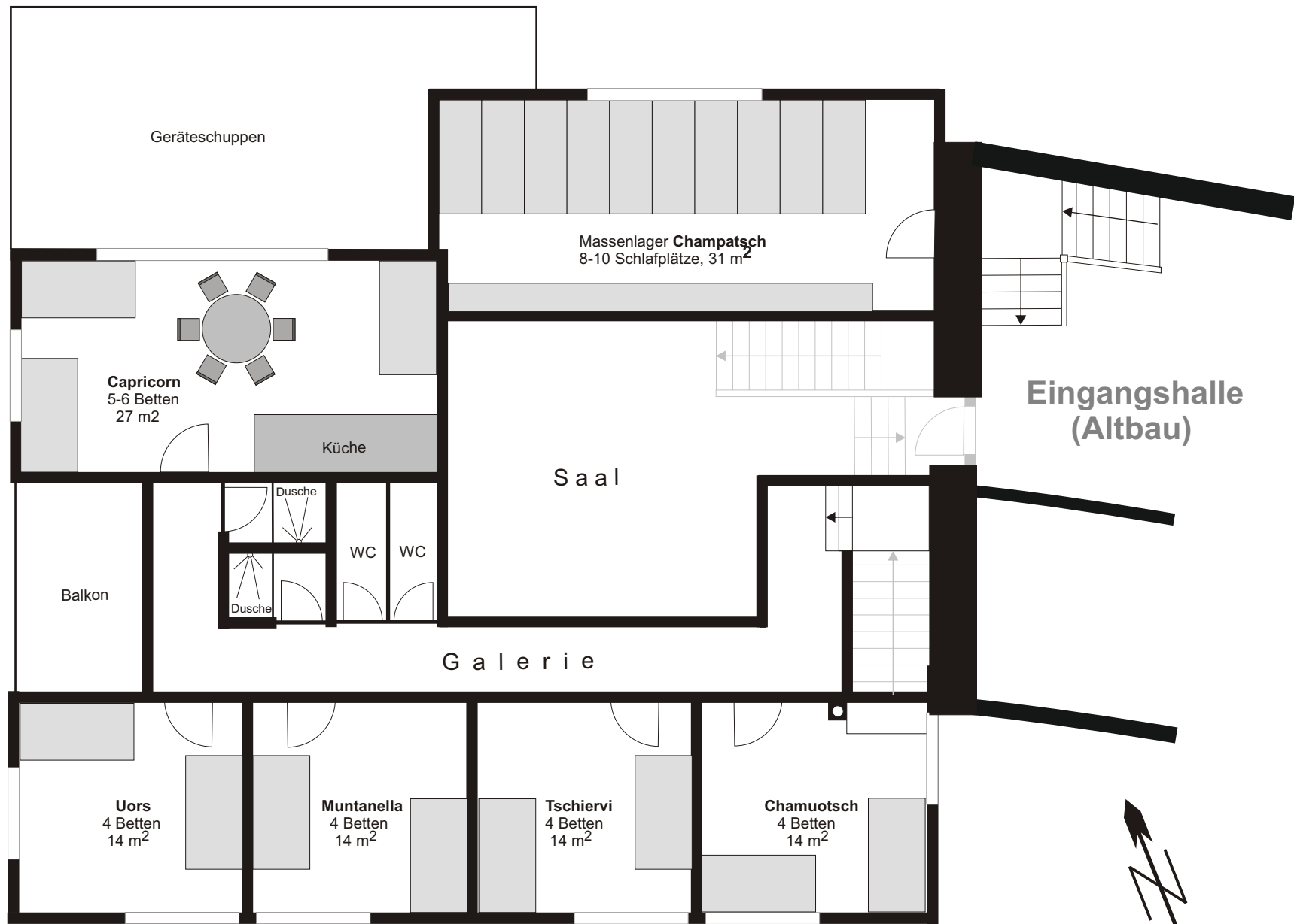
Zimmerplan Obergeschoss (Neubau)
