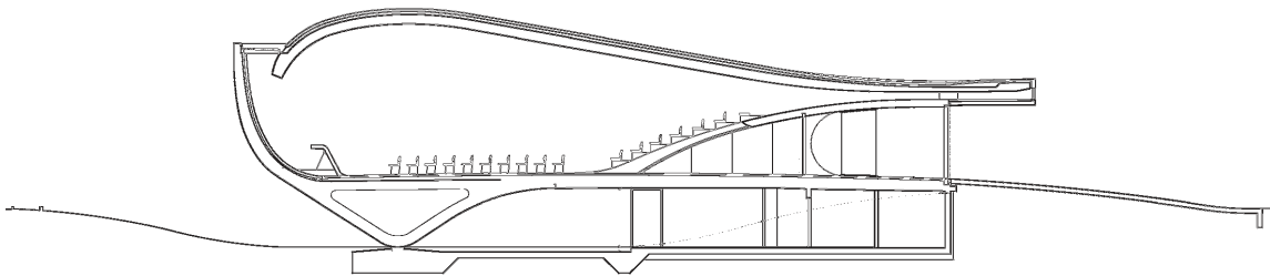
Längsschnitt
