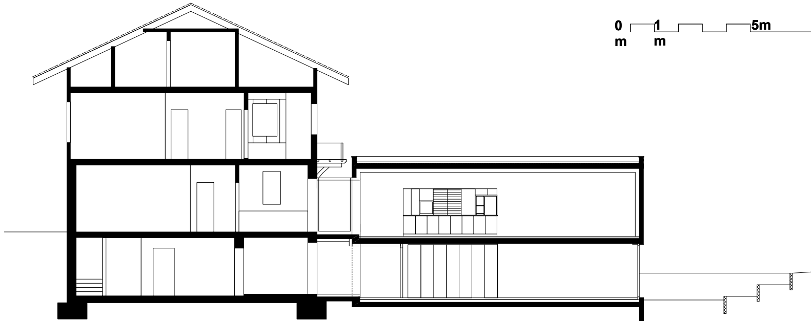
SCHNITT A-A
