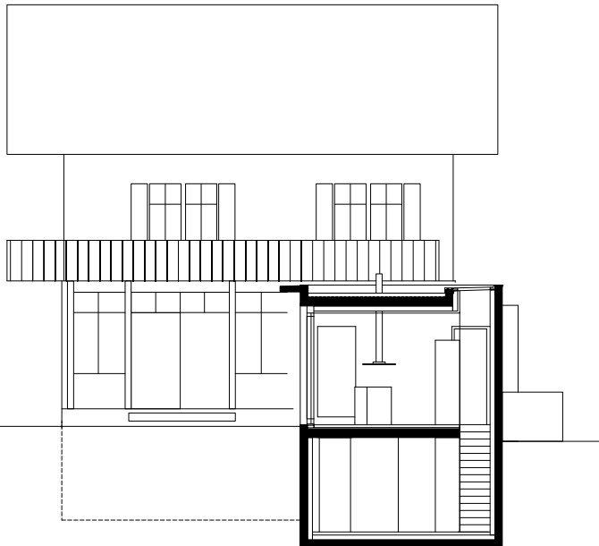
SCHNITT B-B
