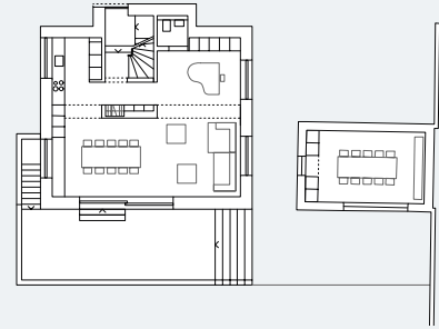
Erdgeschoss
