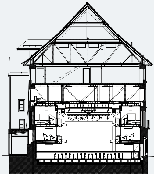
Querschnitt
