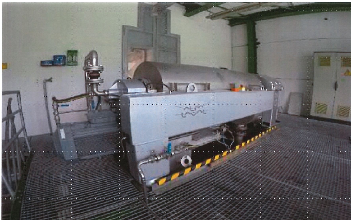
Dekanter ZSA Pfannenstiel
