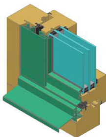
Das Holz-Metallfenster lichtoptimiert
