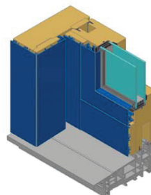
Hebeschiebetüren Holz + Holzmetall
