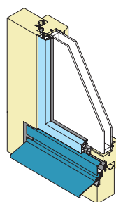
Das bewährte Flügelabdecksystem für Holzfenster überzeugt durch filigrane Ansichtsbreiten.
