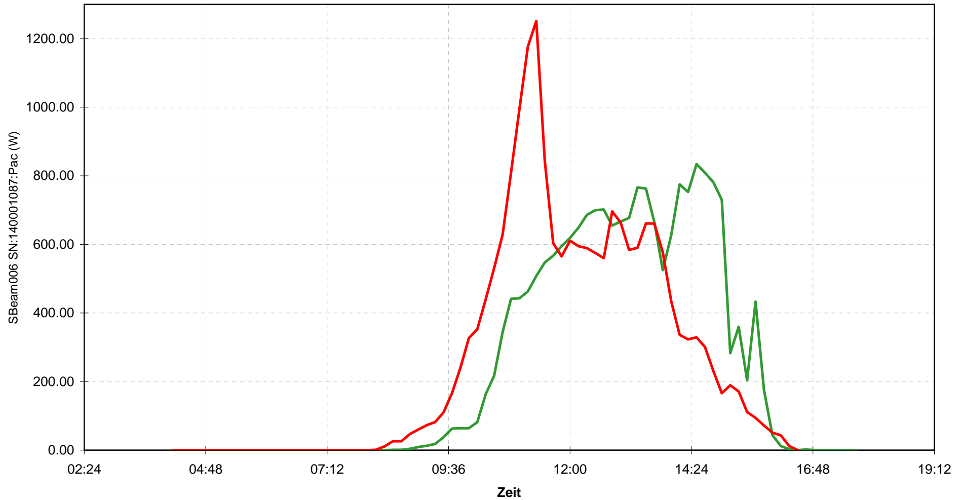
Meßdaten der Photovoltaikanlage vom 26.11.2005 und 27.11.2005 (Tagesleistungen: 3.26/3.28 kWh) www.posthof.ch
