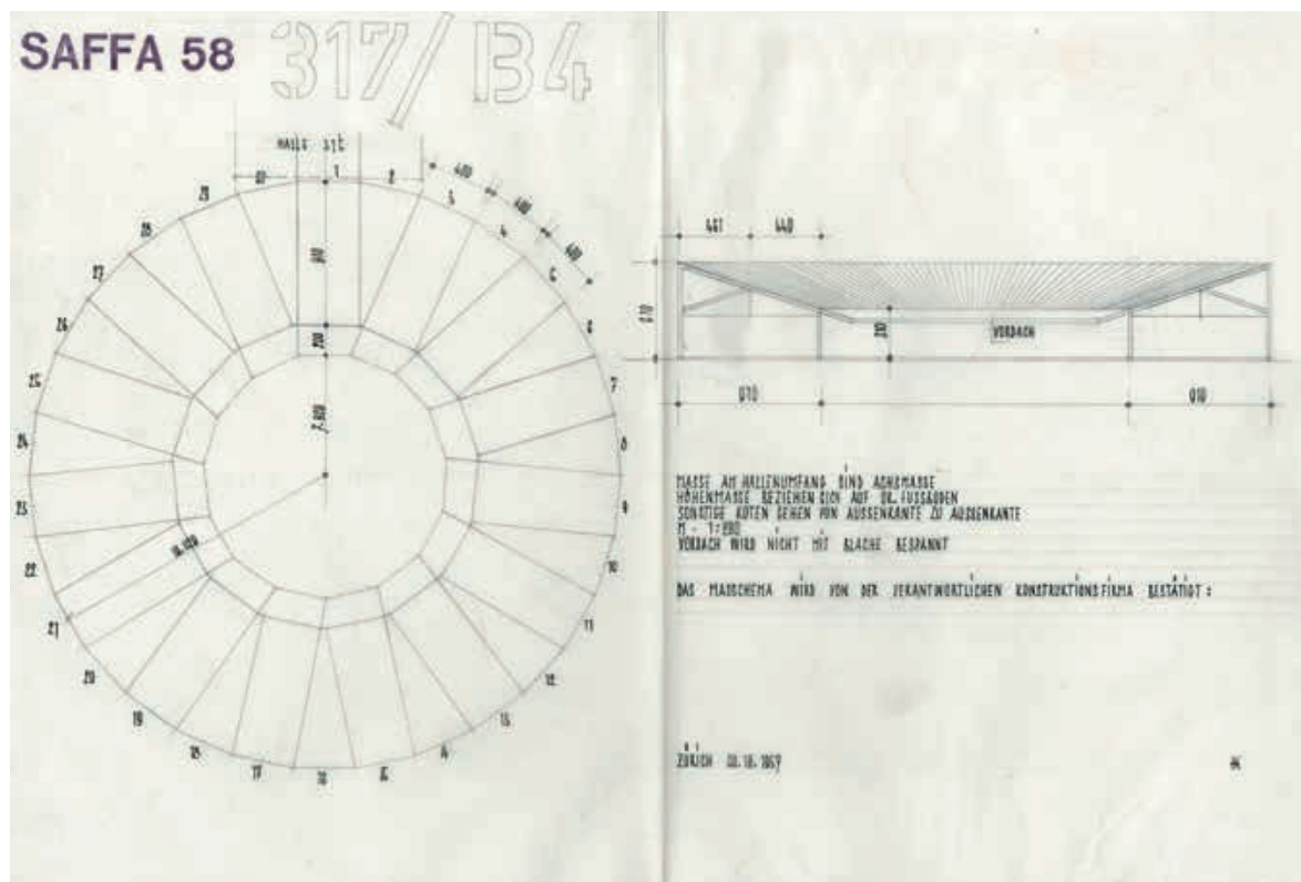
Plan der Rundhalle «Häusliche Erziehung» (gta Archiv)
