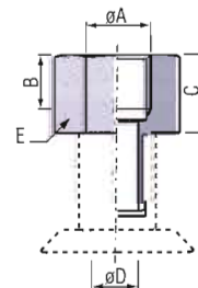
Nippel mit Innengewinde
