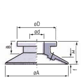
Nippel IM5D6 - IM18D6
