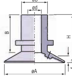
Nippel mit Innengewinde
