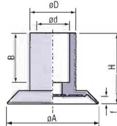
Nippel mit Außengewinde
